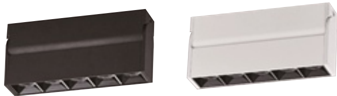
리니얼 B형 5등 직부 LAMP LED 4WX5 CCT 3000k ,4000K, 5700K SIZE 42X202 H94 BEAM ANGLE 24°
